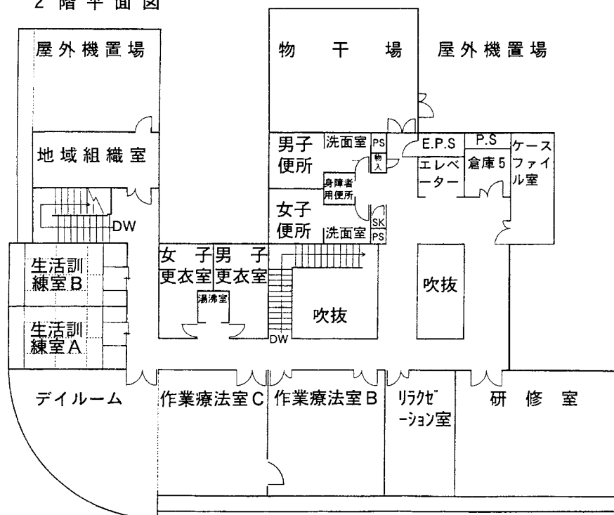
2 階 平 面 図
